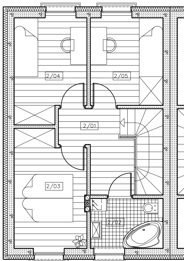
poddasze
